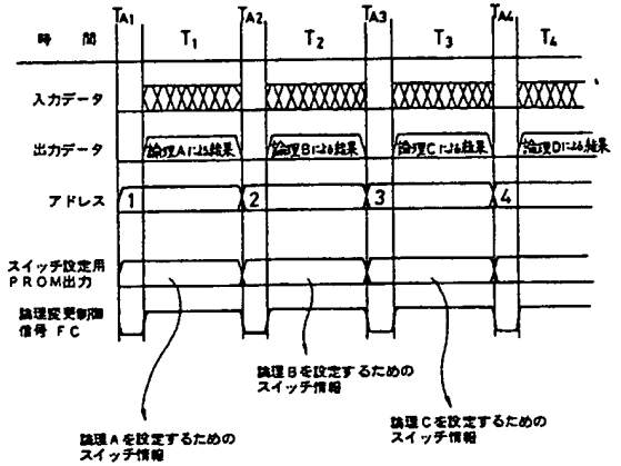
本発明実施例の動作タイミング図 第6図
